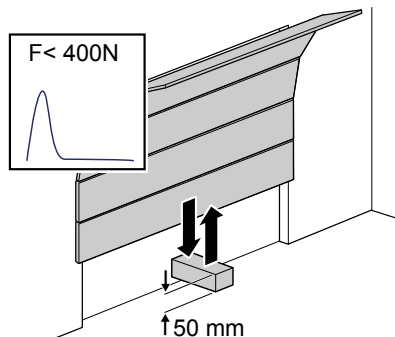
Afb. 7: Krachtbegrenzing controleren
