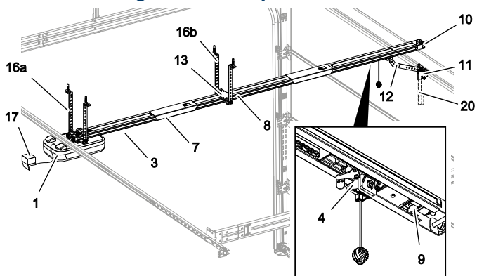
Fig. 1: Panoramica prodotto - Costruito
