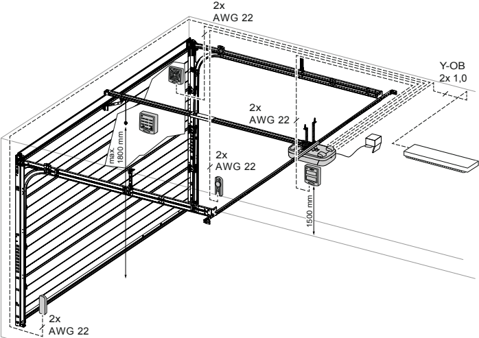
Abb. 3: Beispielinstallation Zubehör
