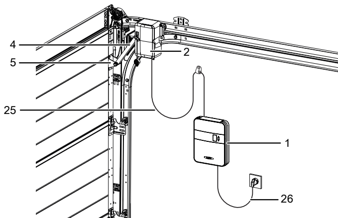
III. 1: Produktoversikt - montert
